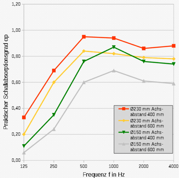
Schallabsorptionsgrad DIN EN ISO 11654 und 354
