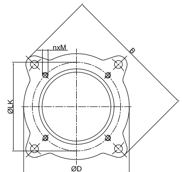
DN 250 - 500
