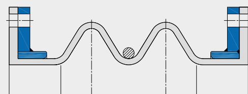
Beispiel - 2-wellig, Ausführung A - unverspannt
