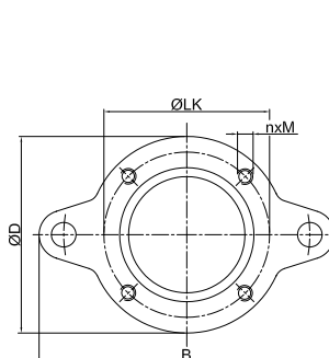
DN 32 - 200
