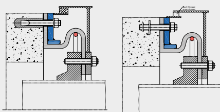
Einbaubeispiel Erdabdeckhaube
